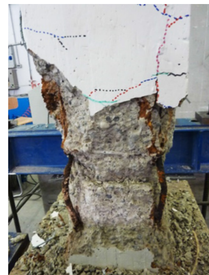
figura 2. Pilastro con armature longitudinali corrose e soggetto a carichi ciclici fino al raggiungimento della rottura per instabilità delle barre longitudinali (Meda, A., Mostosi, S., Rinaldi, Z., Riva, P., "Experimental evaluation of the corrosion influence on the cyclic behaviour of RC columns", Engineering Structures, 76, 2014, 112-123).
