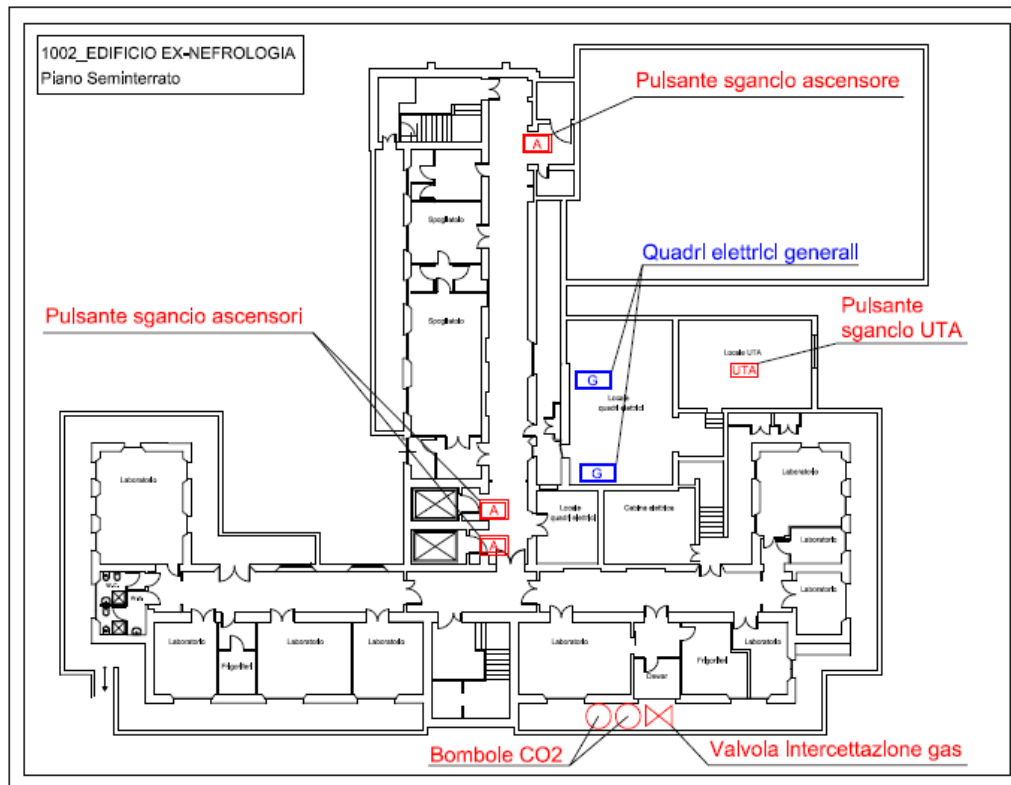
Figura 1. Ubicazione pulsanti sgancio impianti tecnologici .
