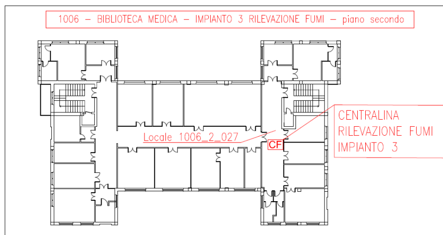
Figura 1.3 - Impianti gestione emergenze – Impianto 3.
