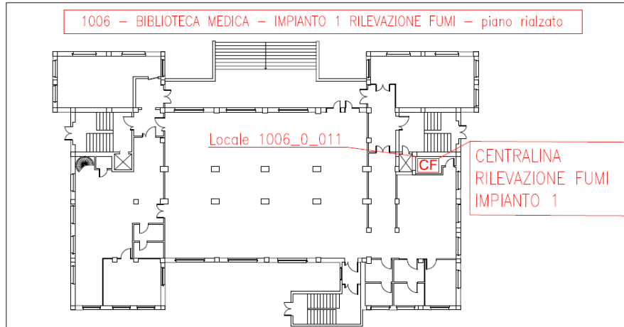
Figura 1.1 - Impianti gestione emergenze – Impianto 1.
