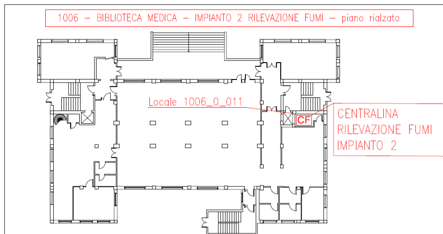
Figura 1.2 - Impianti gestione emergenze – Impianto 2.
