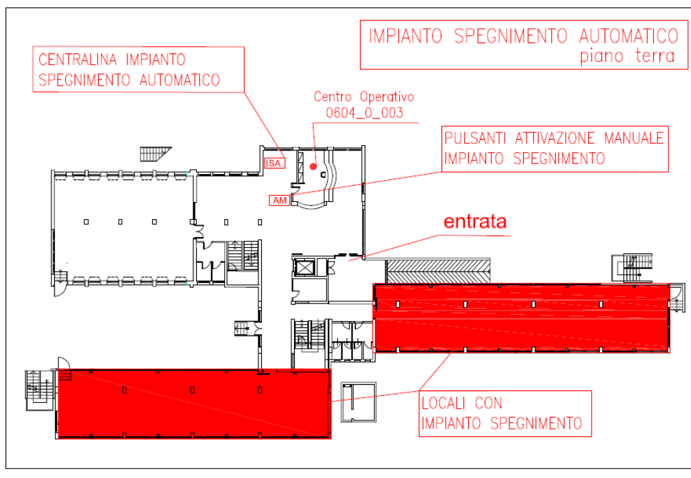
Figura 2 - Impianti spegnimento automatico.
