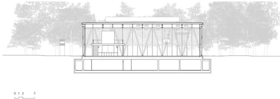
Figura 4 - Sezione trasversale
