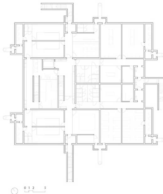
Figura 3 - Piano interrato
