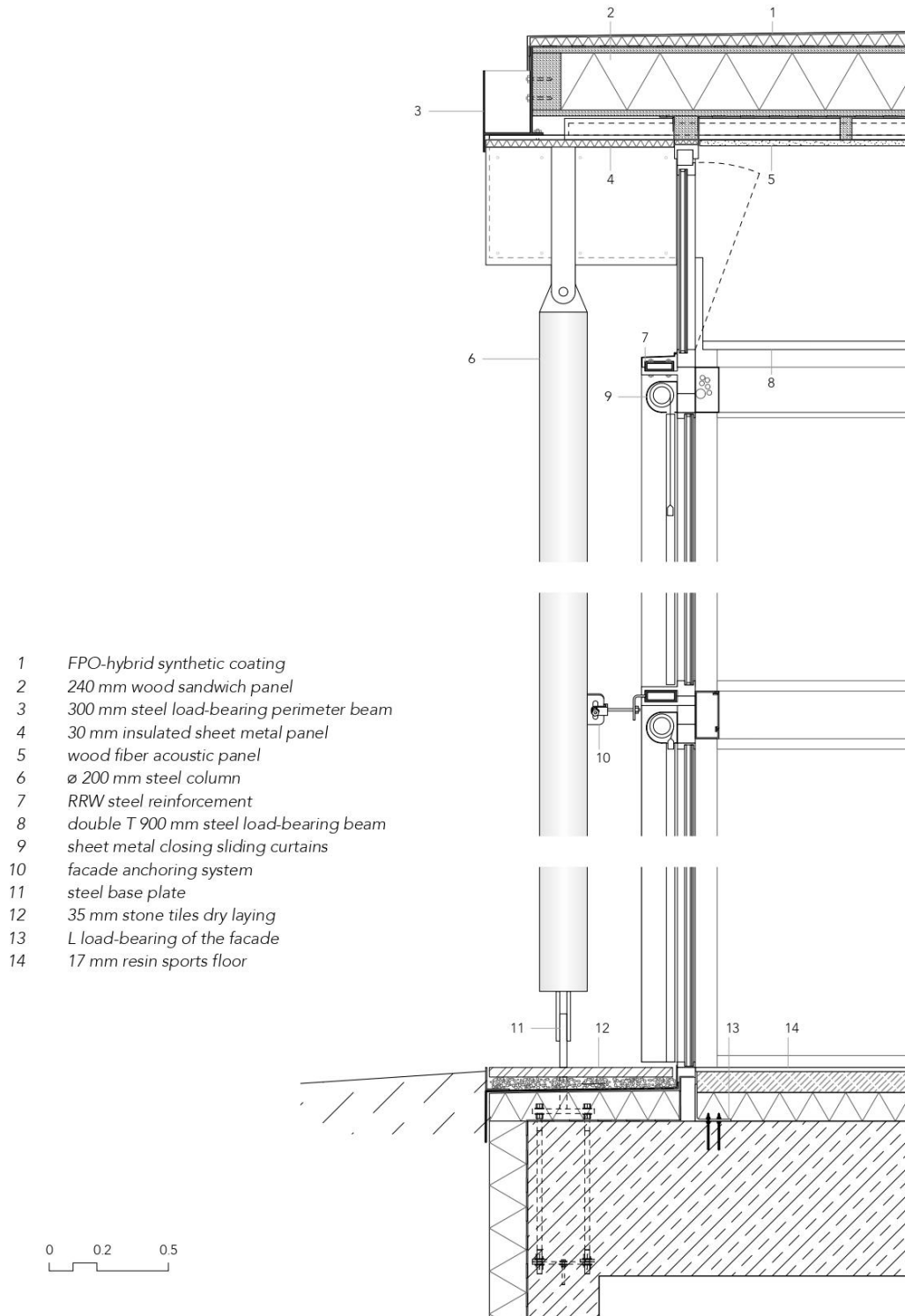
Figura 7 - Particolare costruttivo della facciata
