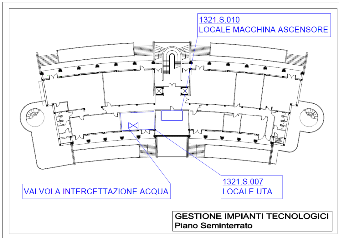
Figura 2.1 Gestione impianti tecnologici – piano seminterrato
