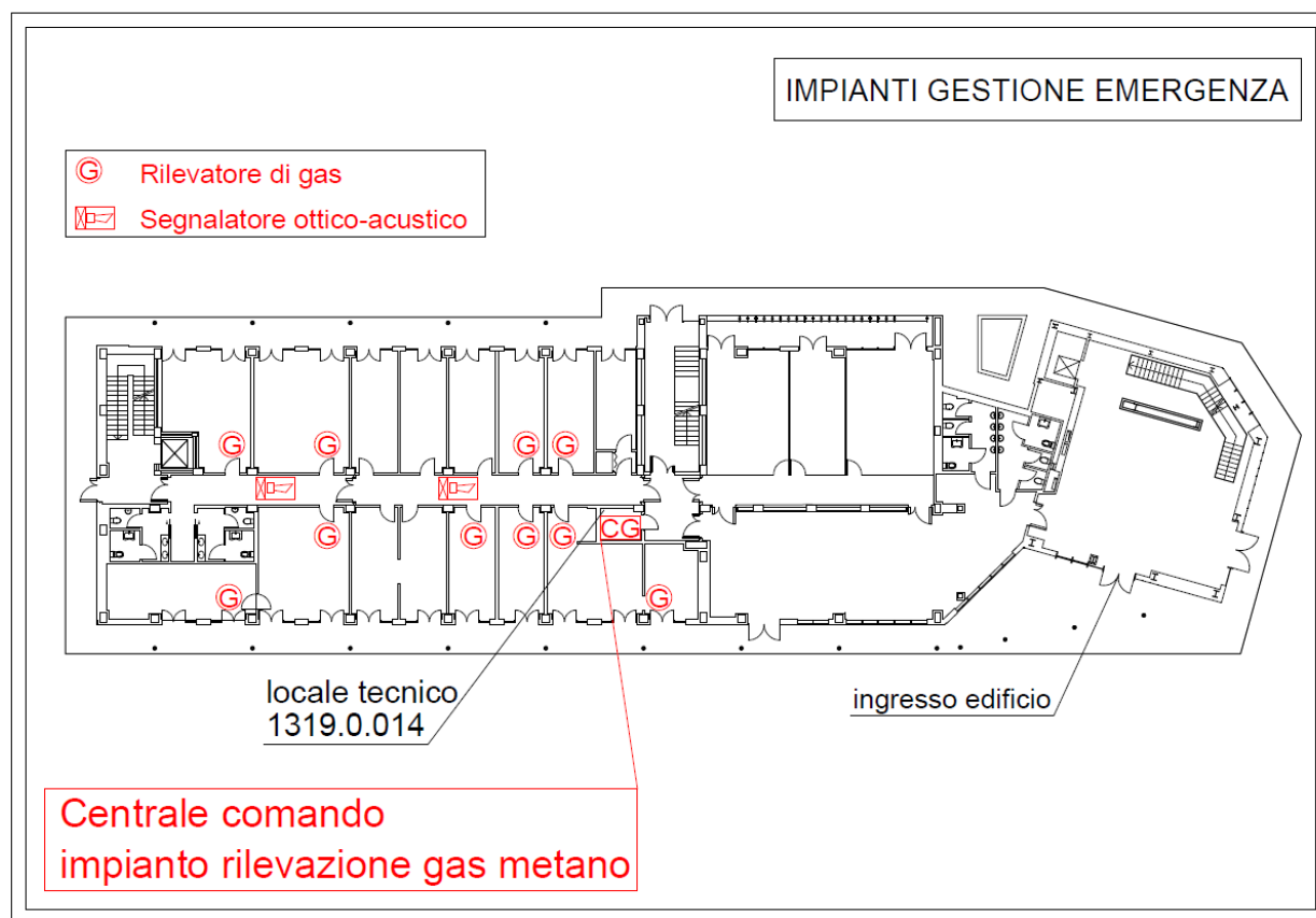
Figura 2 - Impianti rilevazione gas metano e butano
