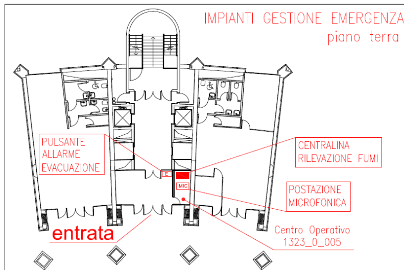
Figura 1. Impianti gestione emergenze.
