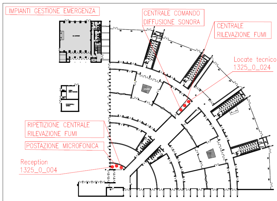
Figura 1 - Impianti gestione emergenze – Piano Terra.
